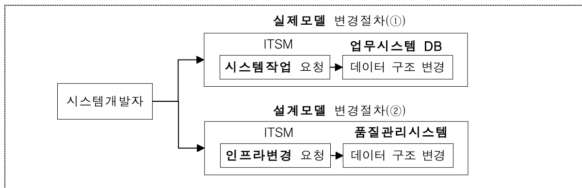
[그림 3] 데이터 설계모델과 실제모델의 변경 절차
